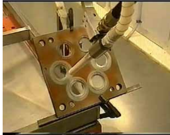
Automatische Reinigung mit mehrachsigem Roboter
